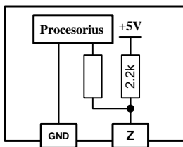
Įėjimo ekvivalentinė schema
