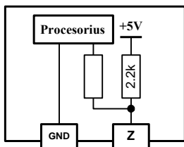
Įėjimo ekvivalentinė schema
